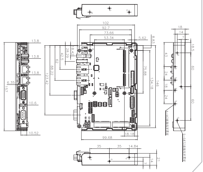
WAFER-BT-i1
